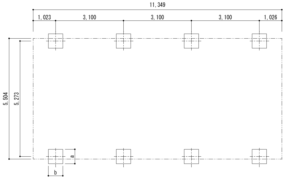
■基礎配置図
